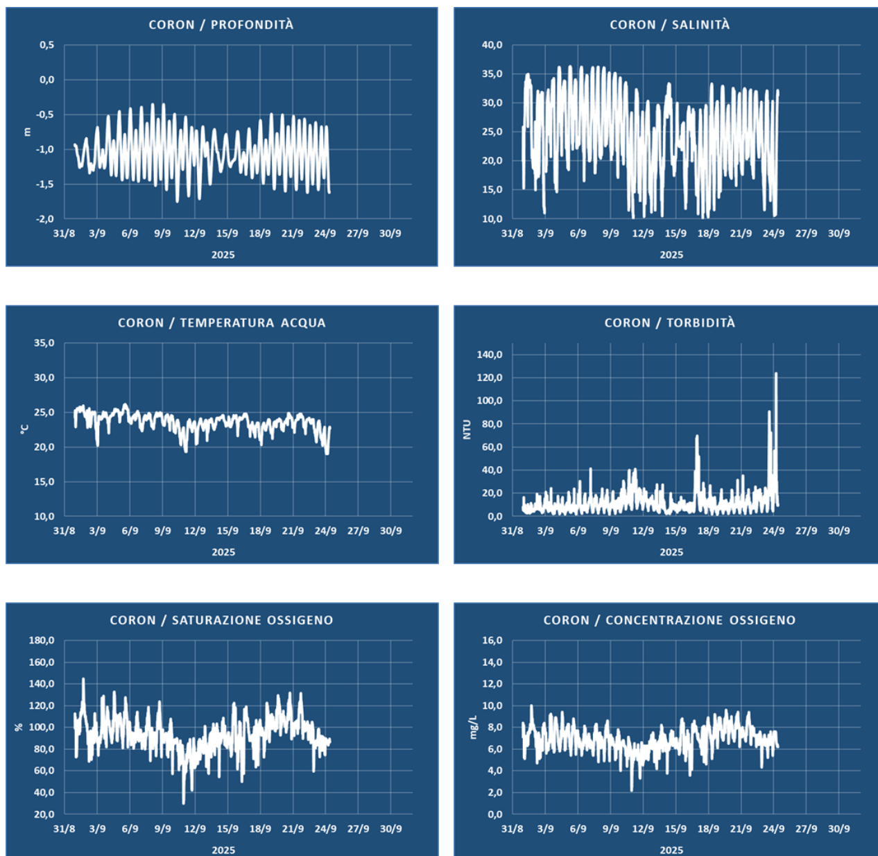
Figura 2: Misure idrologiche e di torbidità
