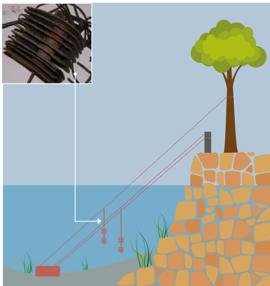
Schema di come i supporti artificiali possono essere fissati tramite cima a strutture (es. albero). In alto a sinistra: foto dei supporti artificiali formati da lamelle di faesite riunite insieme tramite viti e distanziate da gommini a formare dei grappoli ad area definita.
