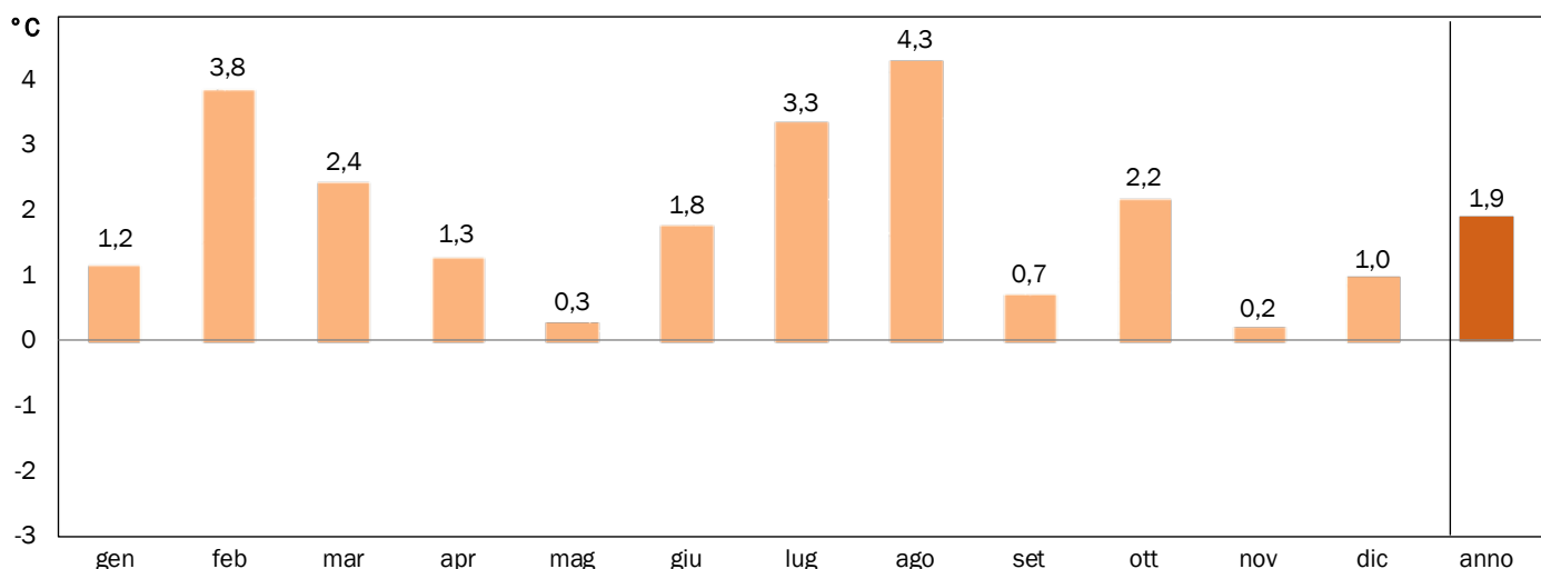
Anomalia delle temperature medie mensili del 2024 a Udine rispetto al periodo 1901-2023 (serie HistAlp 1901-1991, RAFVG 1992-2024).
