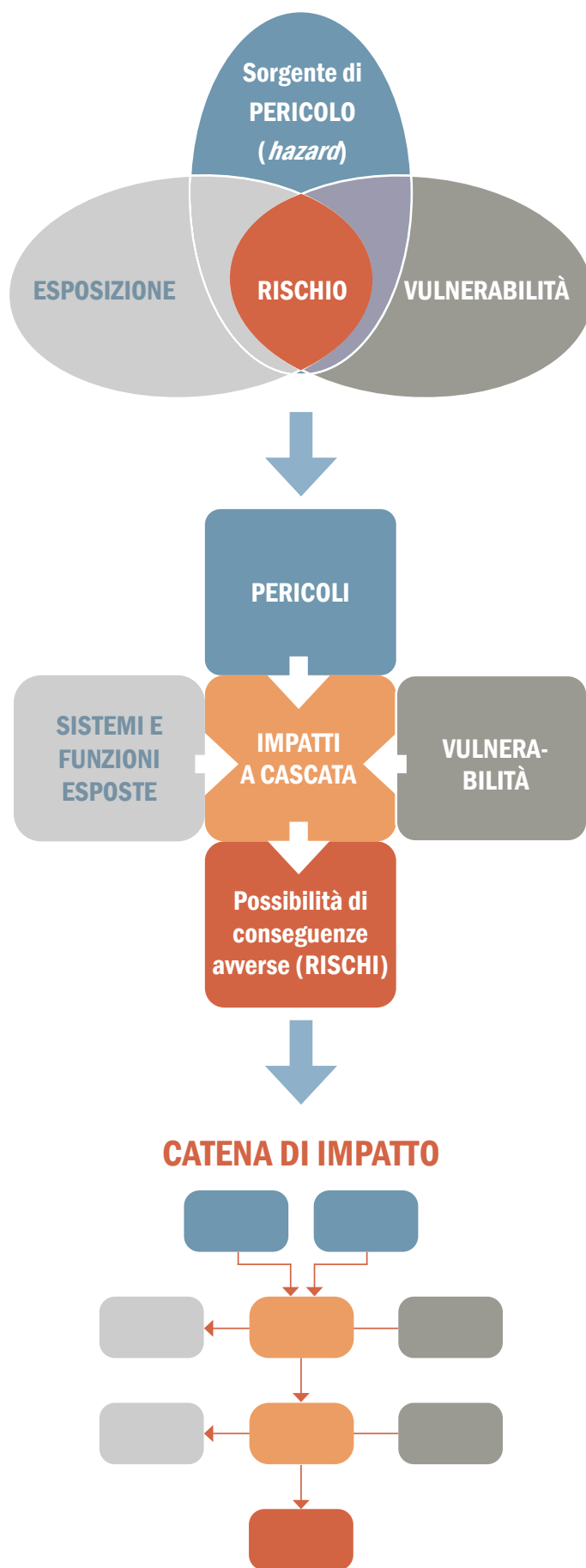
In alto: concetto di rischio e suoi determinanti (IPCC 2021).
