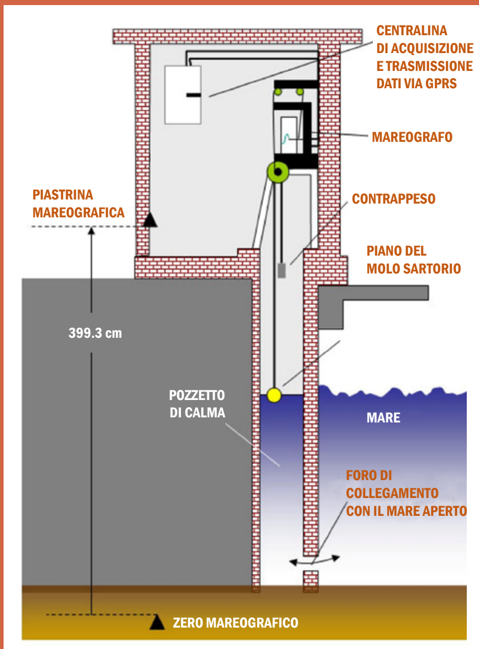
Sezione della cabina mareografica del Molo Sartorio (Trieste).
