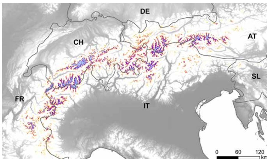
Carta della distribuzione del permafrost nelle Alpi (progetto Permanet https://www.permanet-alpinespace.eu/home.html ).
