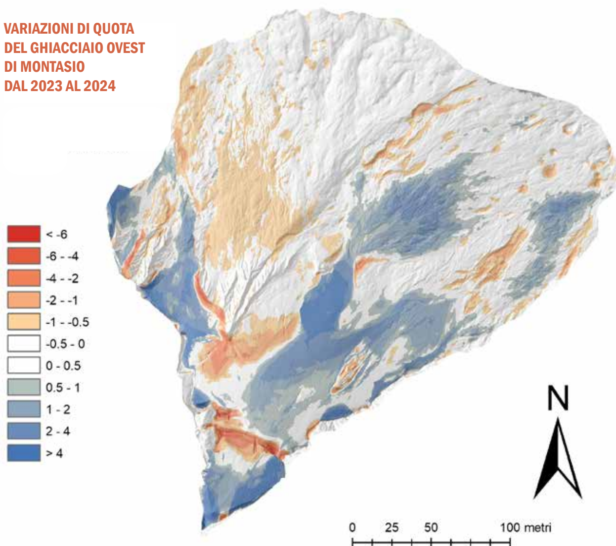
Variazioni di quota (m) della superficie del ghiacciaio occidentale di Montasio tra il 3 ottobre 2023 e il 1 ottobre 2024.
