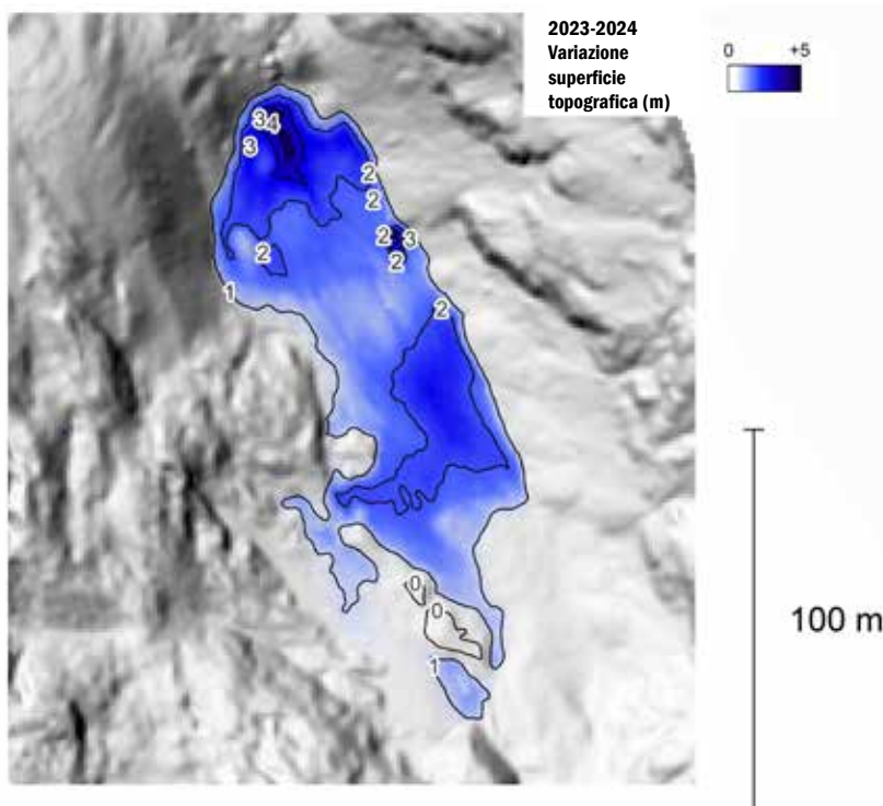
Variazioni di quota (m) della superficie del corpo glaciale orientale del Canin tra il 3 ottobre 2023 e il 1 ottobre 2024.
