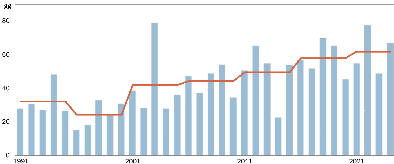
Il grafico rappresenta il numero di giorni caldi (Tmax > 30 °C, istogrammi azzurri) mediato su 14 località rappresentative dell'intera pianura regionale (Brugnera, Capriva del Friuli, Cervignano del Friuli, Cividale del Friuli, Codroipo, Fagagna, Gemona del Friuli, Gradisca d'Isonzo, Palazzolo dello Stella, Pordenone, San Vito al Tagliamento, Talmassons, Udine e Vivaro). La linea arancione rappresenta la media quinquennale.
