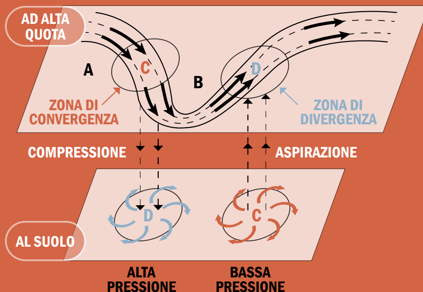
Corrente a getto in quota e formazione di cicloni e anticicloni al suolo*.
