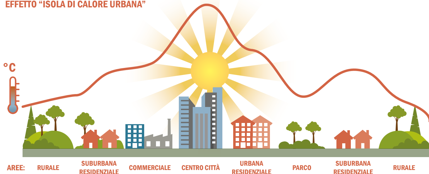
Schema generale dell'effetto "isola di calore urbana" (rielaborato e tradotto da https://community.wmo.int/en/activity-areas/urban/urban-heat-island ).
